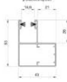
prowadnica kątowna
