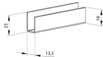
prowadnica przestrzenna
